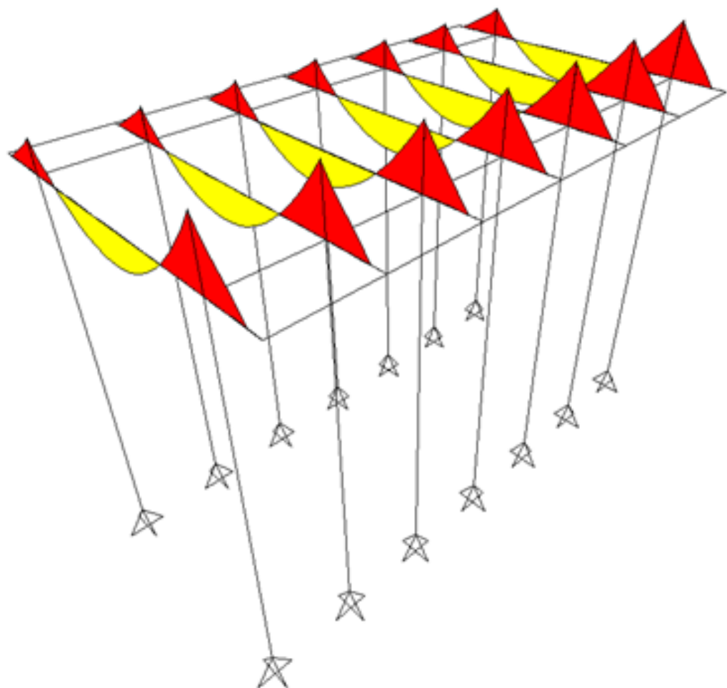
Momento fletor nas vigas devido ao peso próprio das lajes.
