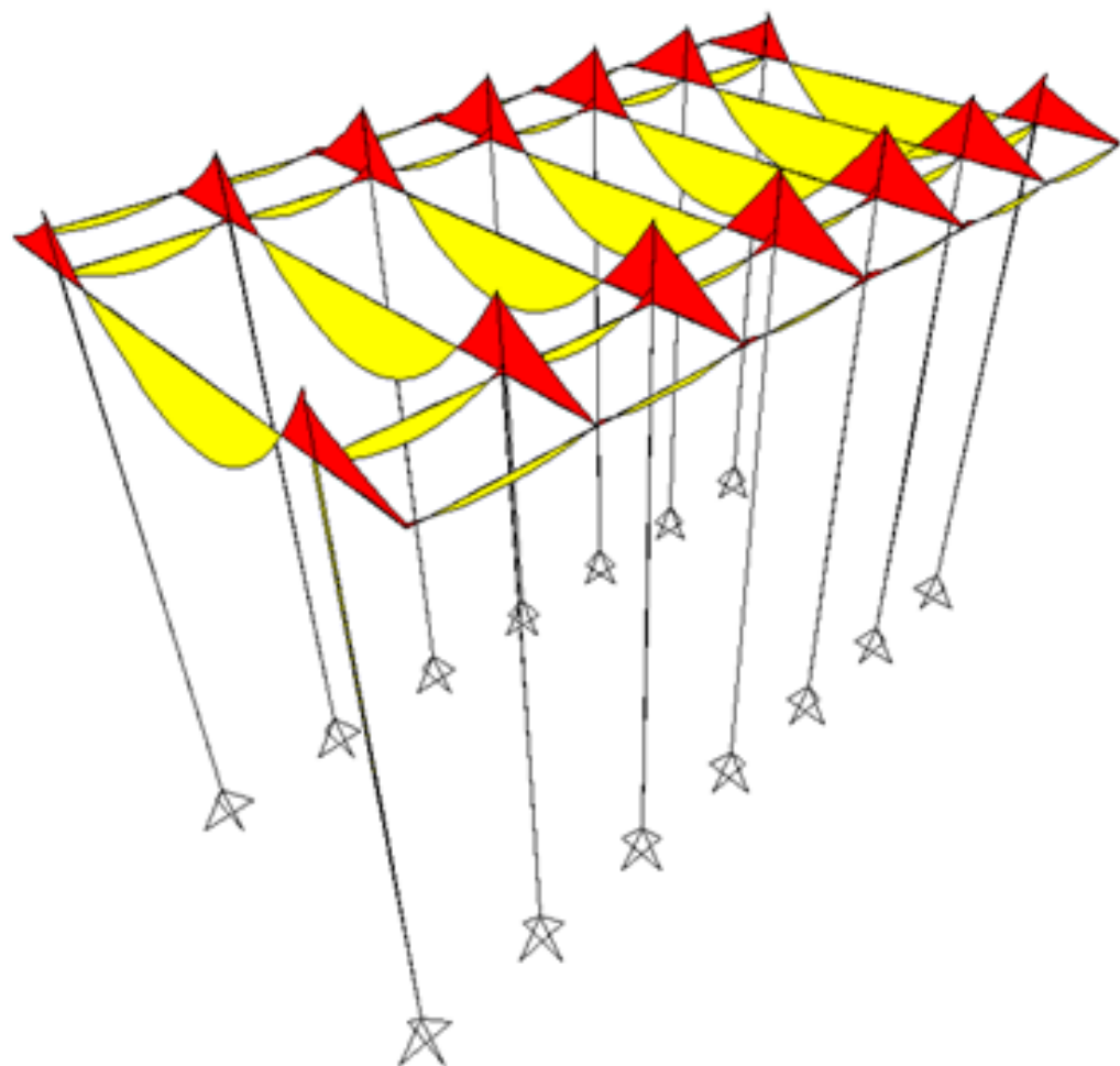
Momento fletor nas vigas devido ao peso próprio das vigas.
